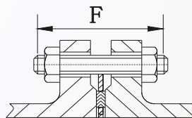
Length of Stud Bolt
