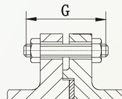
Length of Stud Bolt
